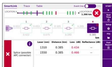
Smart Link Mapper (SLM) Ansicht mit vereinfachter symbolbasierter Darstellung der OTDR-Testergebnisse
