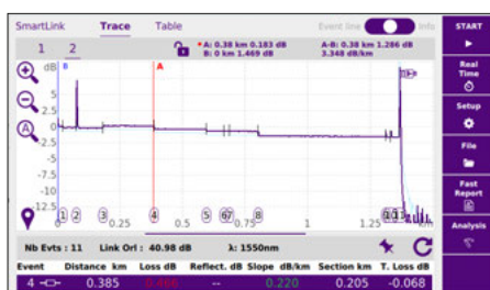
OTDR-Kurvenansicht zur Expertenanalyse und für zusätzliche manuelle Messungen
